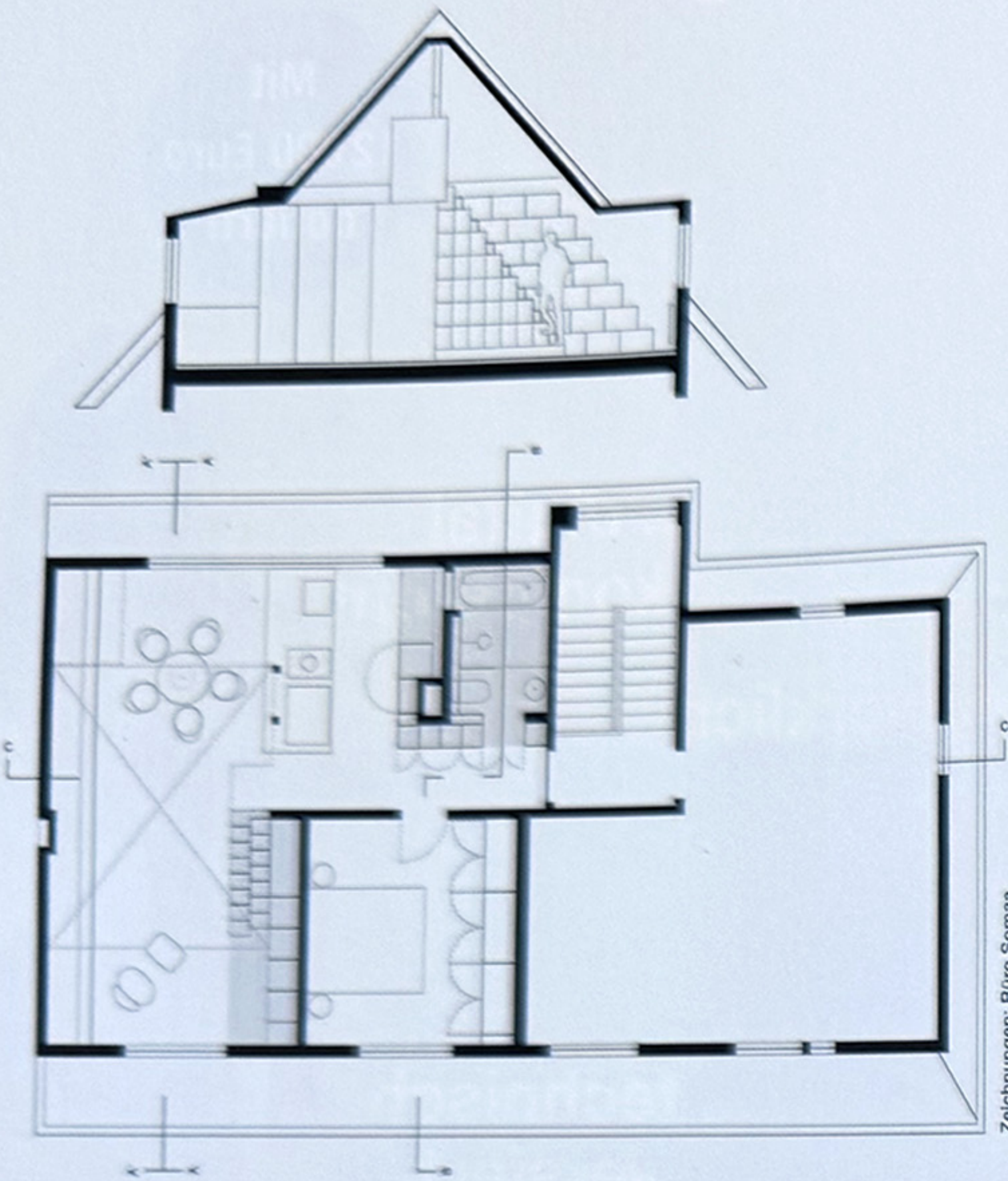
Grundriss und Schnitt der Dachgeschosswohnung mit einem Treppenregal in den Spitzgiebel
